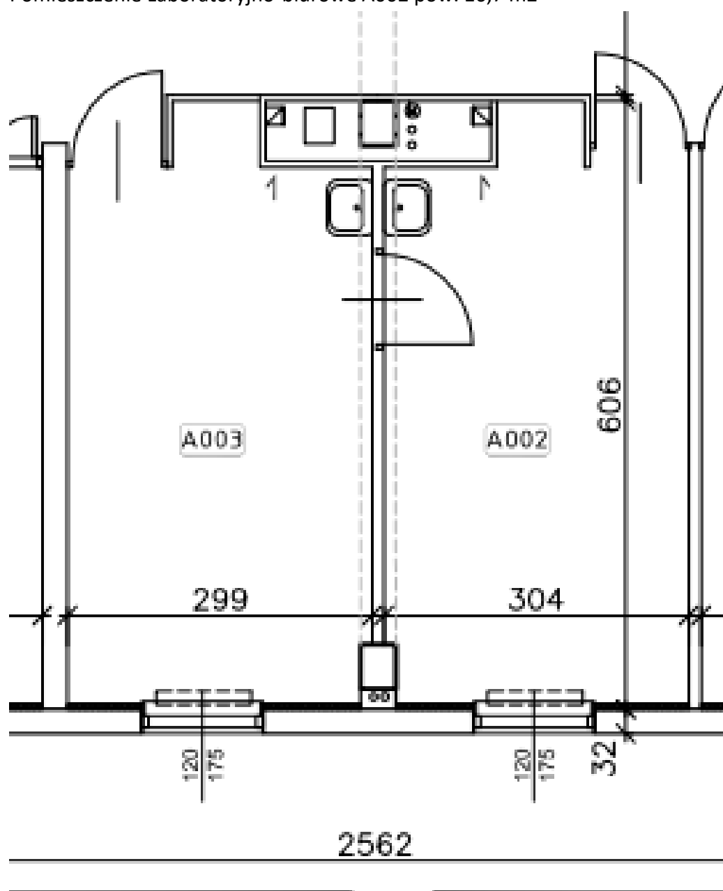
Pomieszczenie Laboratoryjno-biurowe A002 pow. 16,7 m 2
